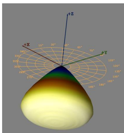
3D разпределение на светлинен поток
