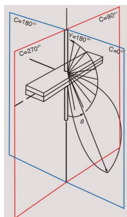
3D разпределение на светлинен поток
