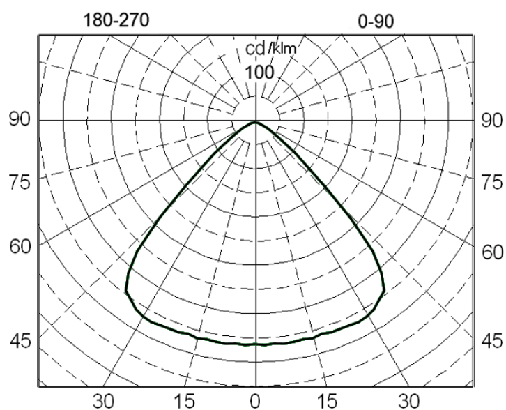
Светлоразпределение при условен светлинен поток 1000lm
