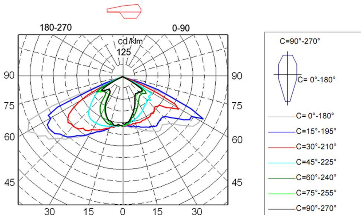
Светлоразпределение при условен светлинен поток 1000lm
