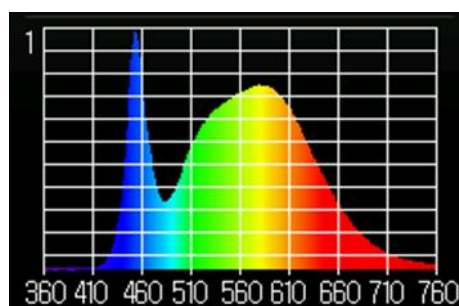
Спектър на светлинен поток 5000K
