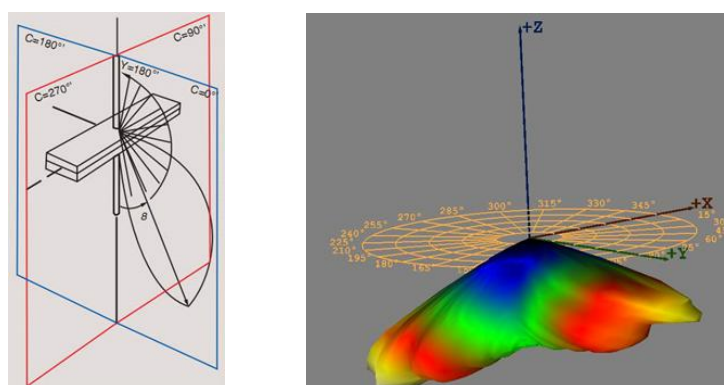
3D разпределение на светлинен поток
