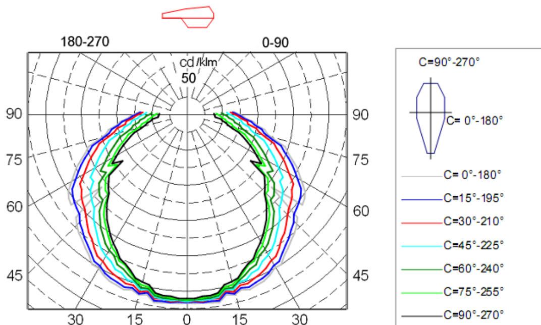
Светлоразпределение при условен светлинен поток 1000lm
