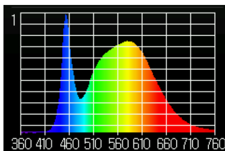
Спектър на светлинен поток 5000K
