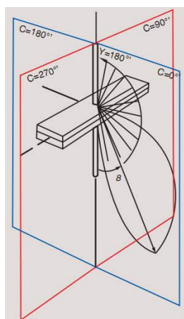
3D разпределение на светлинен поток
