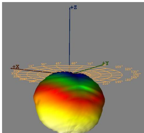
3D разпределение на светлинен поток
